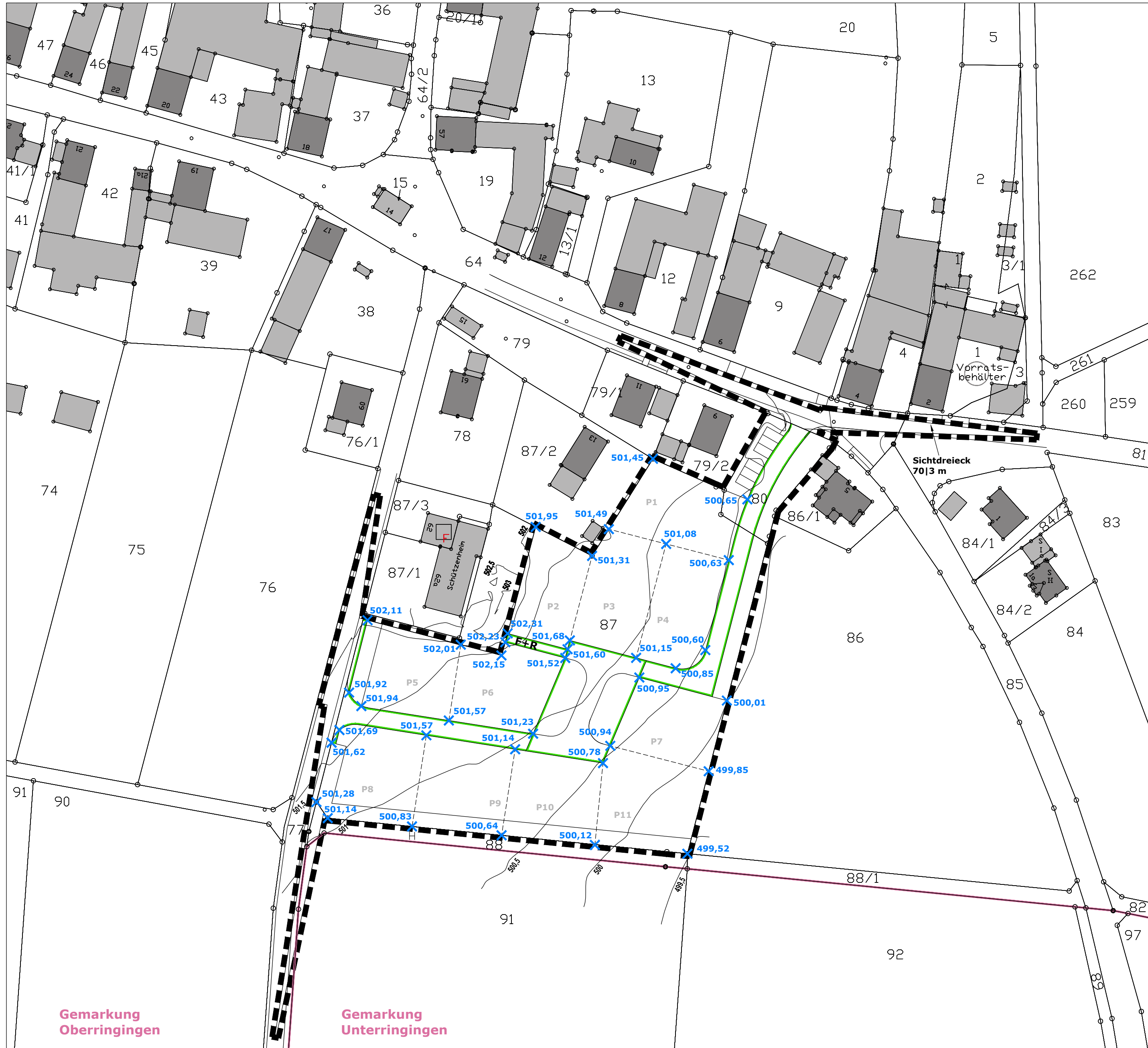
Lageplan mit Festsetzung - Geländehöhen für Parzellen Maßstab 1:1.000
